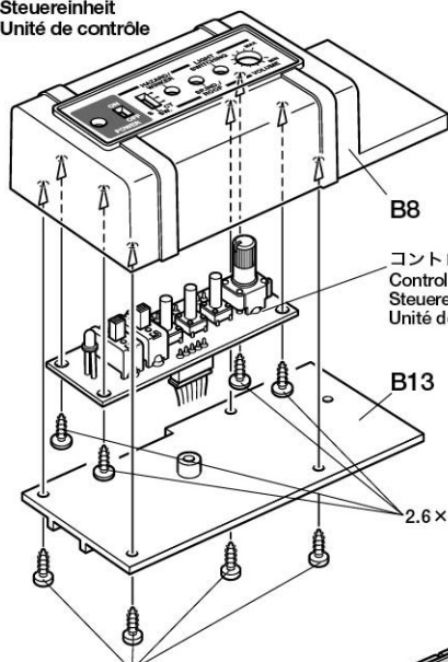
3×8mmタッピングビス Tapping screw Schneidschraube Vis taraudeuse
